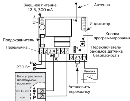
Рис. 1 — Подключение блока автоматики
