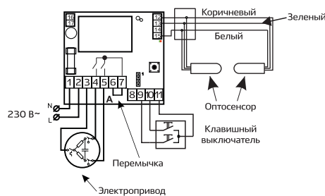
Рис. 2 — Подключение электропривода роллеты и оптоэносора
